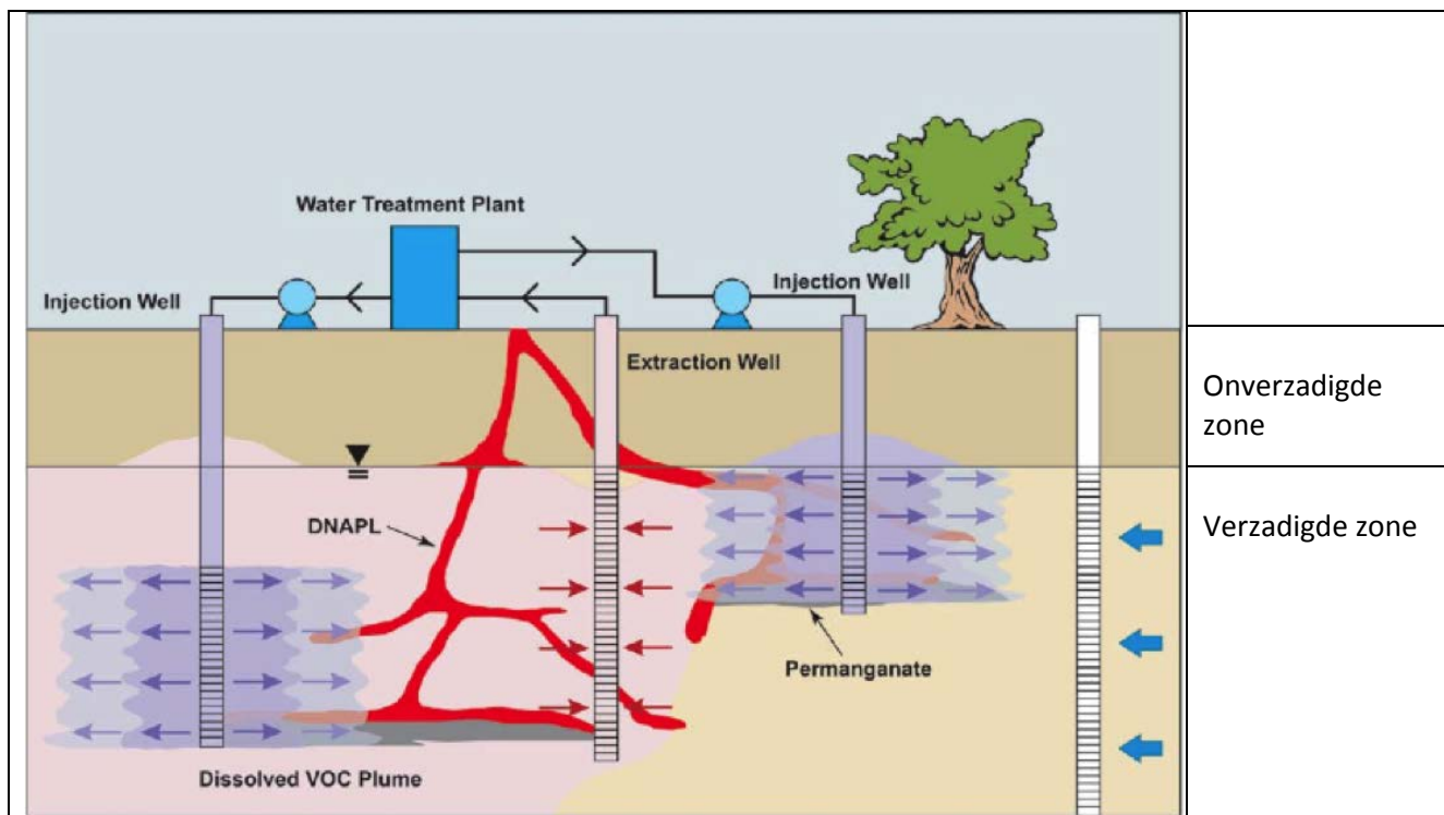
Figuur 2.1- ISCO-regeling
