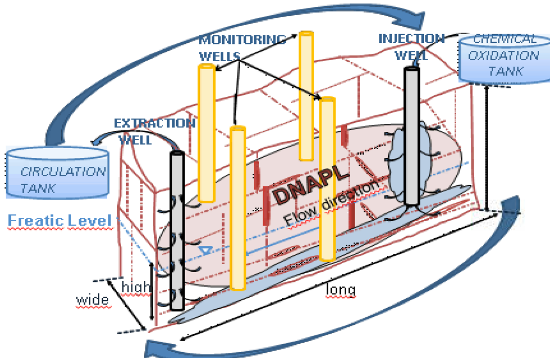
Figuur 2.4- 3D-Recirculatiesysteem
